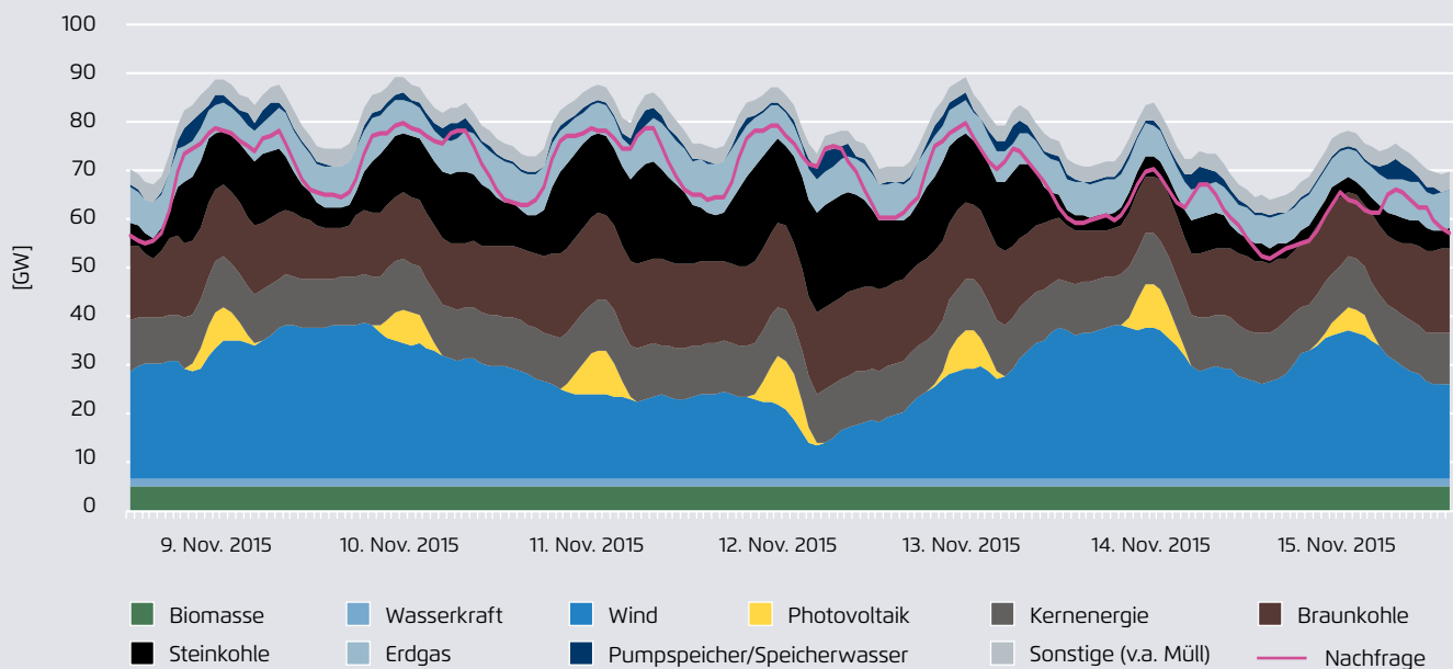
Kalenderwoche 46 mit viel Windstrom und flexiblen thermischen Kraftwerken
