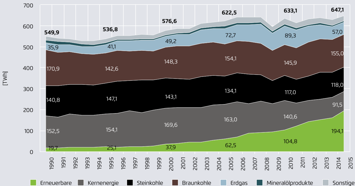
Entwicklung der Stromproduktion: Erneuerbare produzieren 2015 mehr als die Kernenergie in ihren Höchstzeiten Abbildung 2
