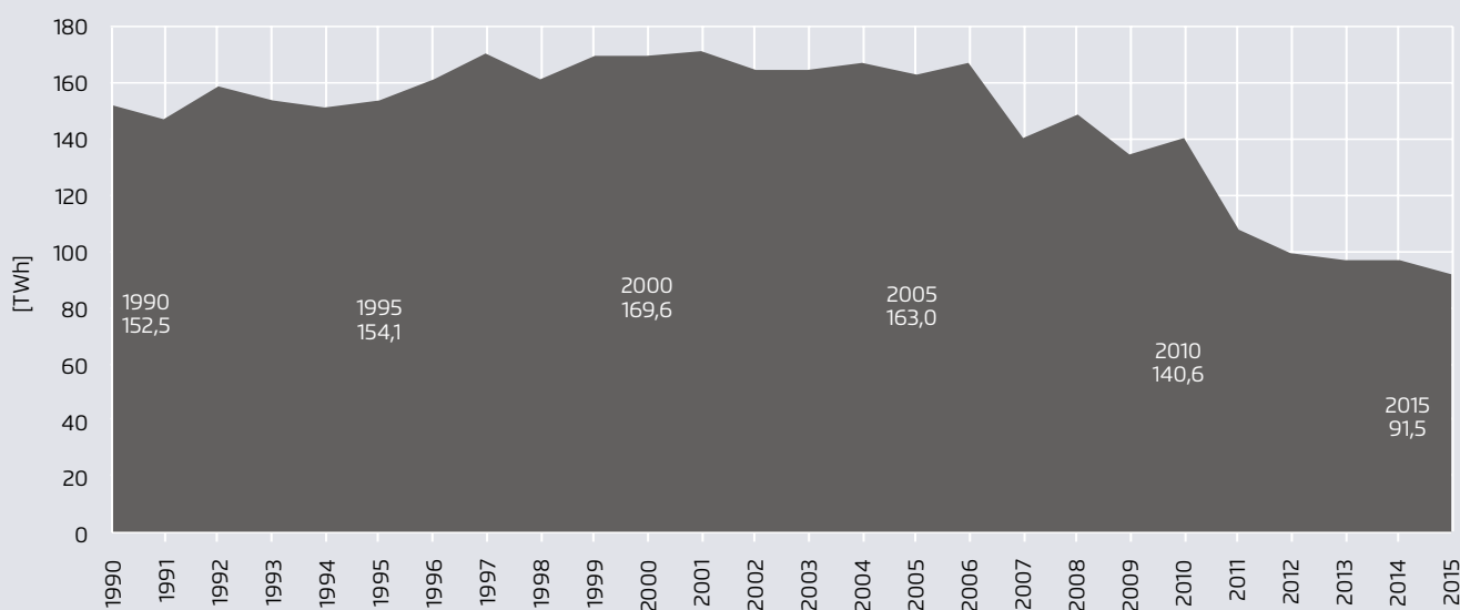
Die Abschaltung des Kernkraftwerks Grafenrheinfeld Ende Juni 2015 macht sich mit einer leicht gesunkenen Stromproduktion bemerkbar: Stromproduktion aus Kernenergie 1990-2015
