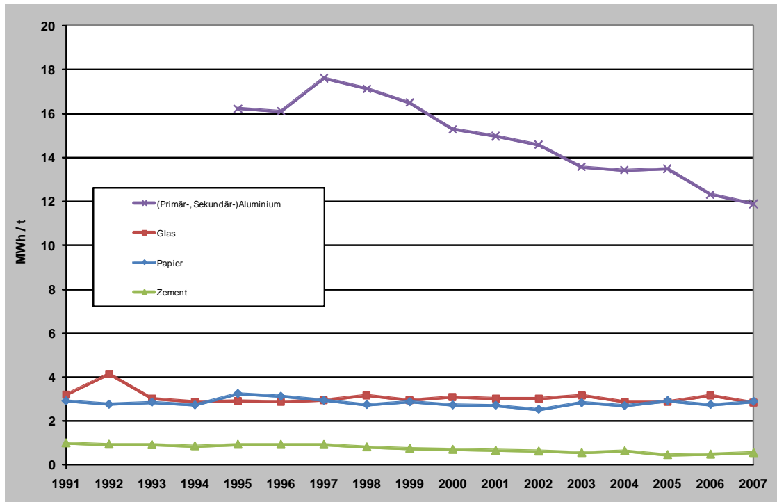
Abbildung 4-14 Entwicklung des Energieverbrauchs pro Tonne einzelner energieintensiver Produkte
