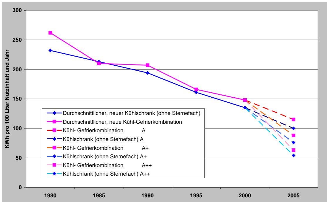
Abbildung 3-8 Entwicklung des jährlichen Stromverbrauchs von neuen Kühlschränken und Kühl-Gefrierkombinationen
