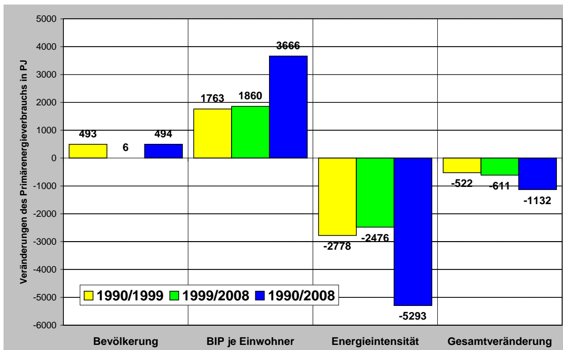
Abbildung 7-5 Beiträge verschiedener Einflussfaktoren zu den Veränderungen des temperatur- und lagerbestandsbereinigten Primärenergieverbrauchs in Deutschland innerhalb der Periode von 1990 bis 2008
