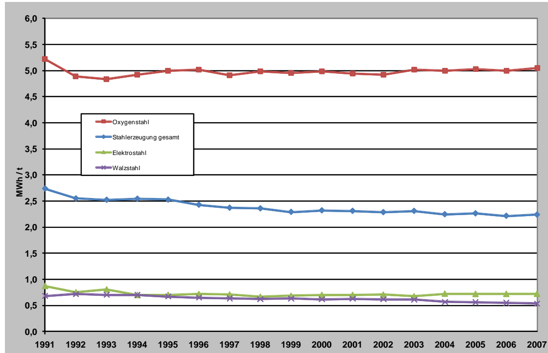
Abbildung 4-13 Entwicklung des Energieverbrauchs pro Tonne Stahl in der Eisen- und Stahlindustrie
