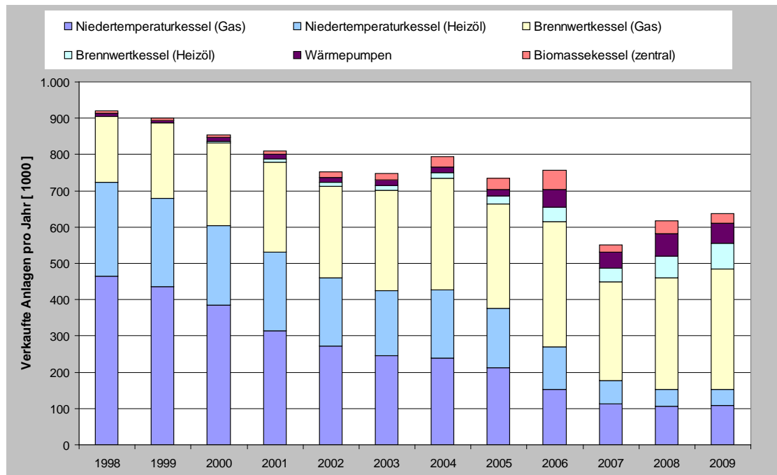
Abbildung 3-21 Absatz an Heizsystemen
