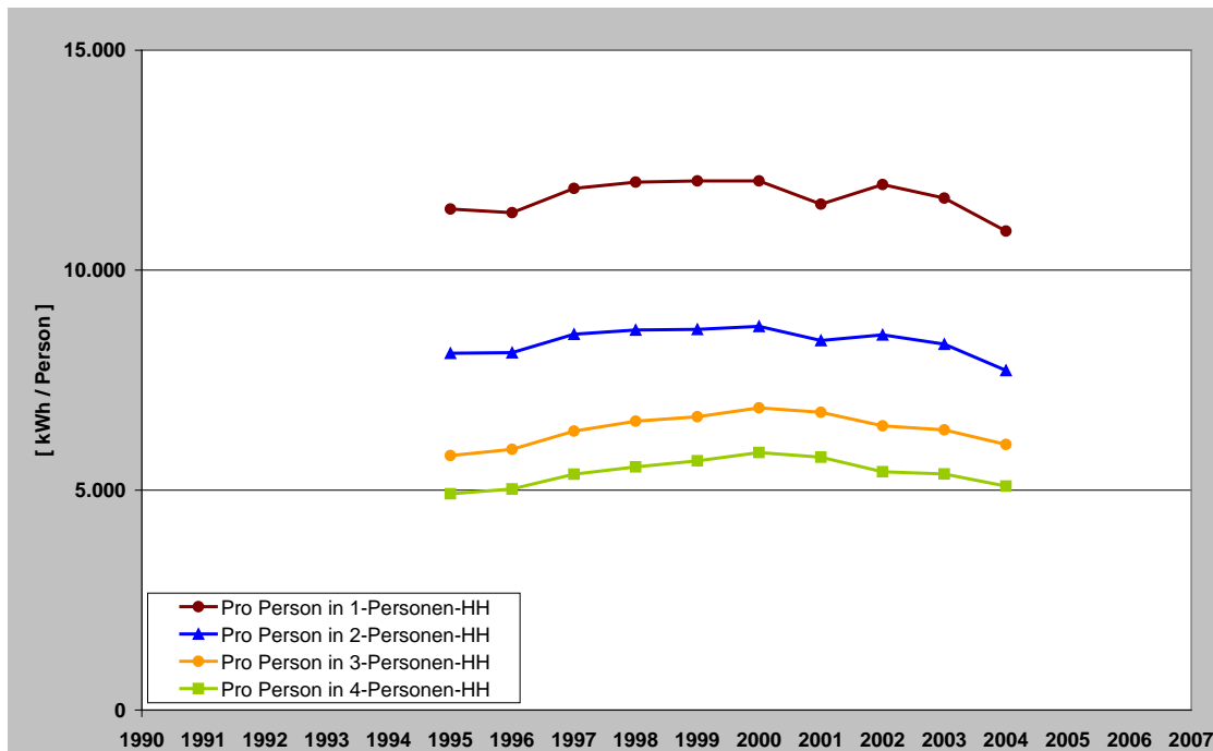
Abbildung 3-13 Endenergieverbrauch für Raumwärme pro Person nach Haushaltsgröße (temperaturbereinigt)
