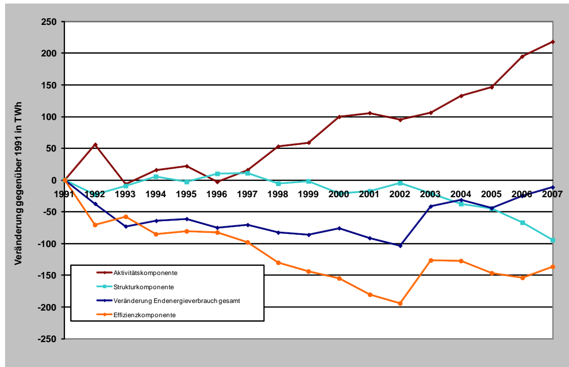
Abbildung 4-7 Komponentenerlegung des Endenergieverbrauchs in der Industrie
