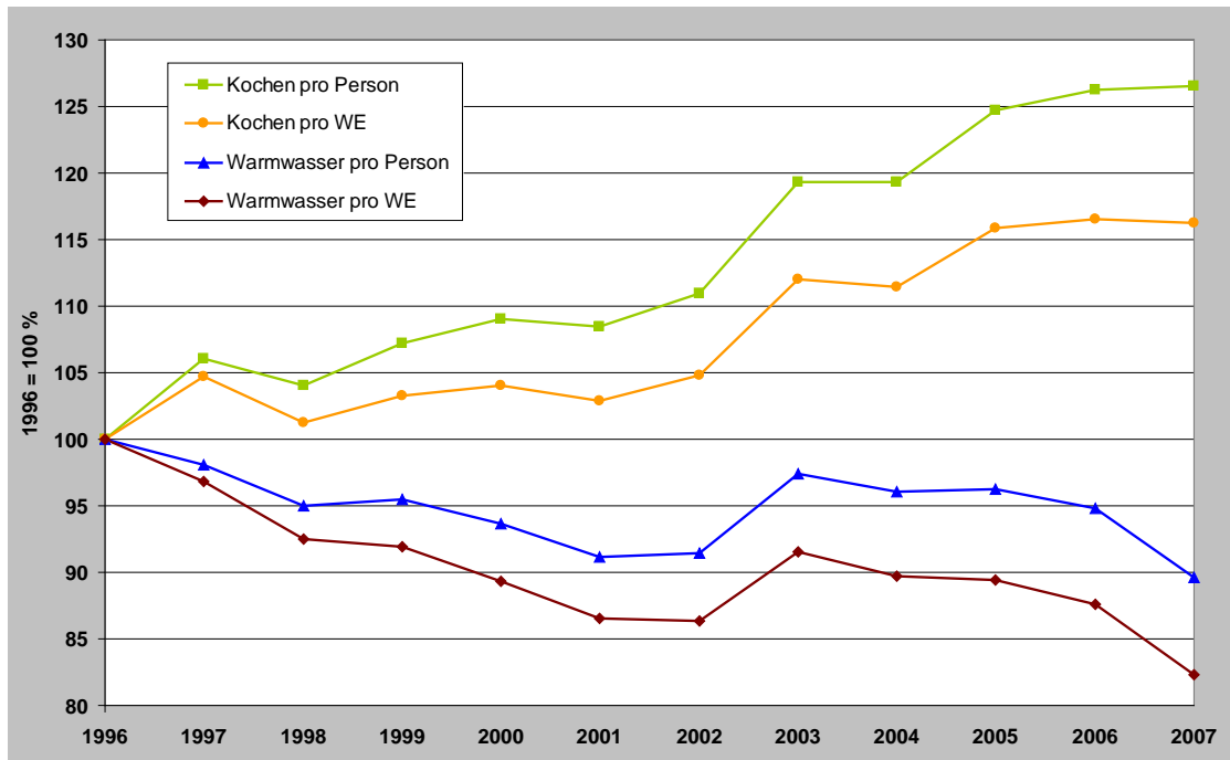
Abbildung 3-15 Entwicklung der spezifischen Energieverbräuche für Warmwasserbereitung und Kochen
