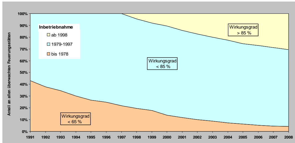
Abbildung 3-22 Altersstruktur und Kessel-Wirkungsgrad der nach 1.BImSchV überprüften Öl- und Gasfeuerungsstätten
