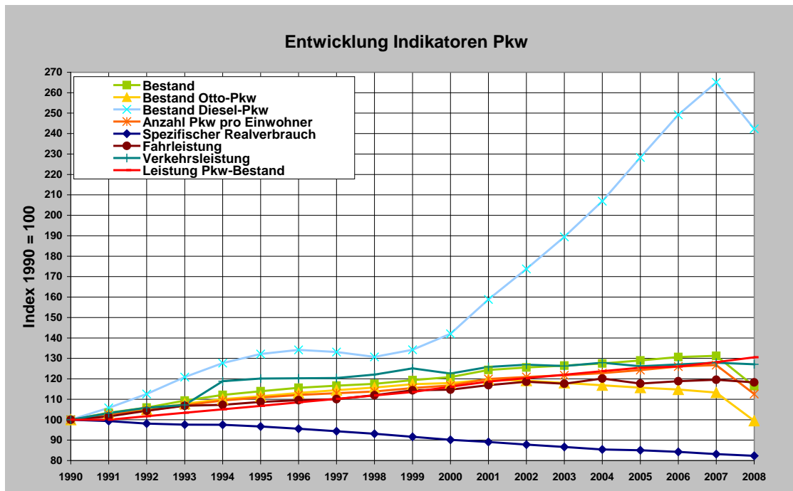
Abbildung 6-10 Entwicklung verschiedener Indikatoren im Pkw-Bestand 37
