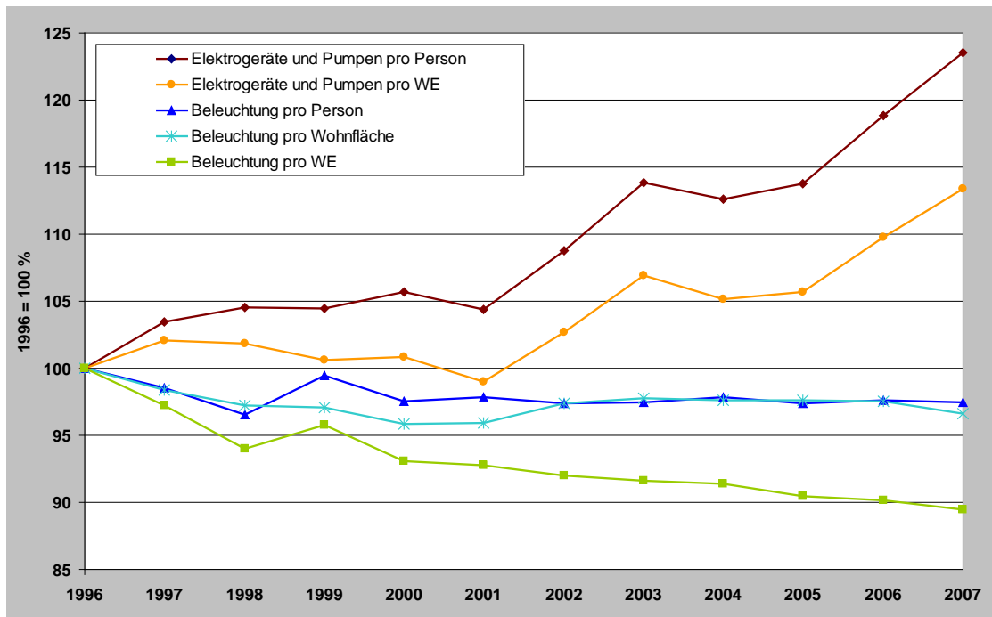
Abbildung 3-16 Entwicklung der spezifischen Endenergieverbräuche für Elektrogeräte und Pumpen sowie Beleuchtung
