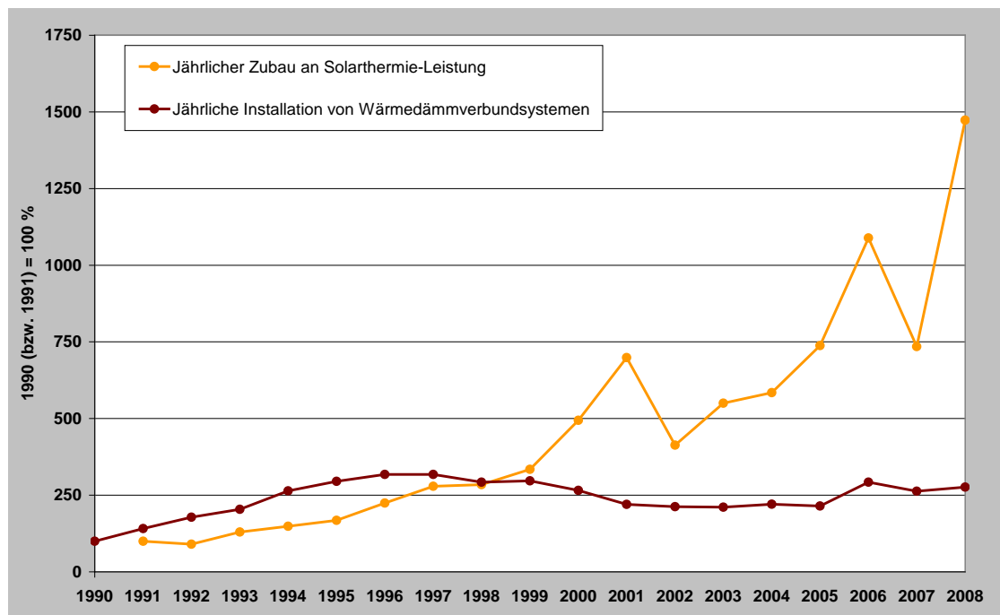
Abbildung 3-23 Zubau von Wärmedämmverbundsystemen und Solarthermie
