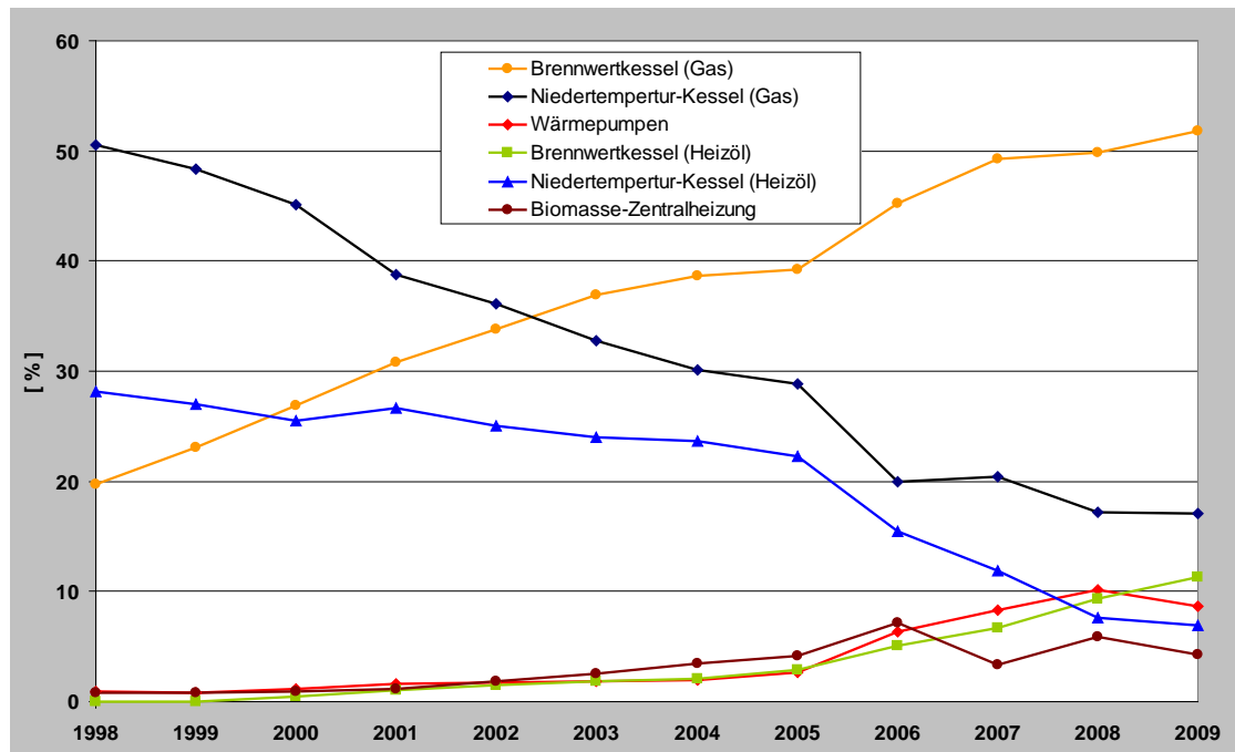
Abbildung 3-20 Anteil der Heizungssysteme am gesamten Absatz
