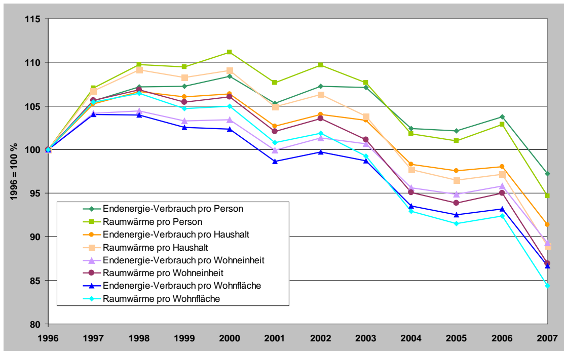
Abbildung 3-12 Vergleich der Indikatoren bezogen auf Gesamt-Endenergiebedarf und Endenergieverbrauch für Raumwärme (jeweils temperaturbereinigt)
